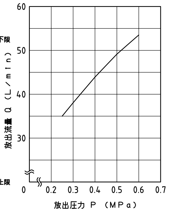
放射量特性 P - Q 曲線
